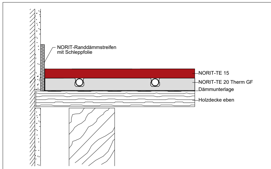
Wandanschluss auf Holzdecke
