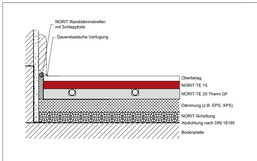
Auf erdberührendem Bauteil
