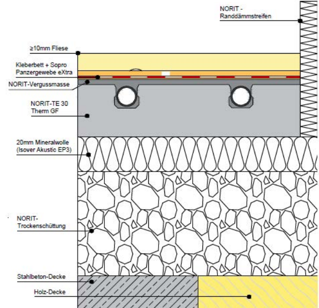
Aufbau 2 – NORIT-TE Therm 30 GF
