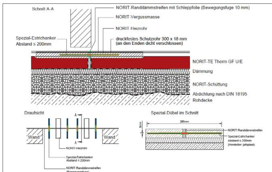
Bewegungsfuge mit Spezial-Estrich-Anker
