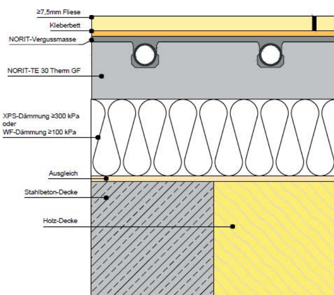
Aufbau 2 – NORIT-TE 30 Therm GF
