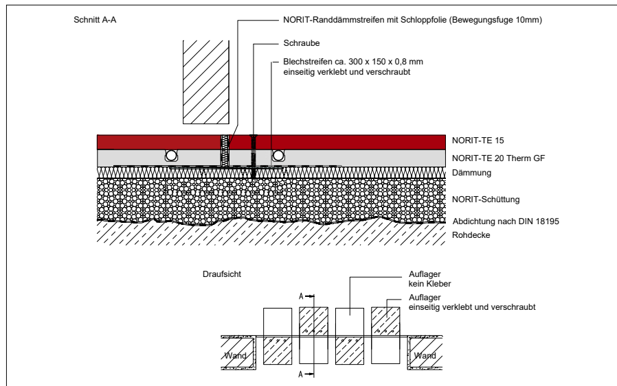
Bewegungsfuge mit Verstärkungsplatte
